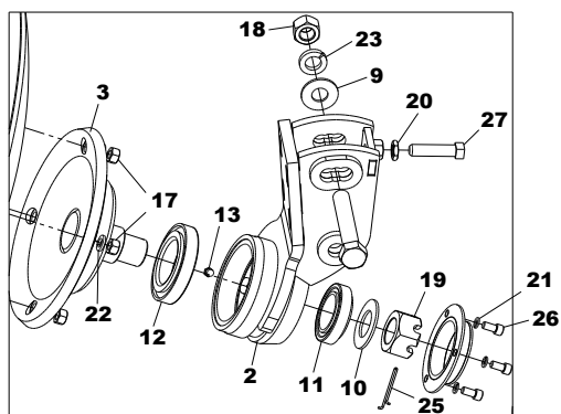
DETALLE A
