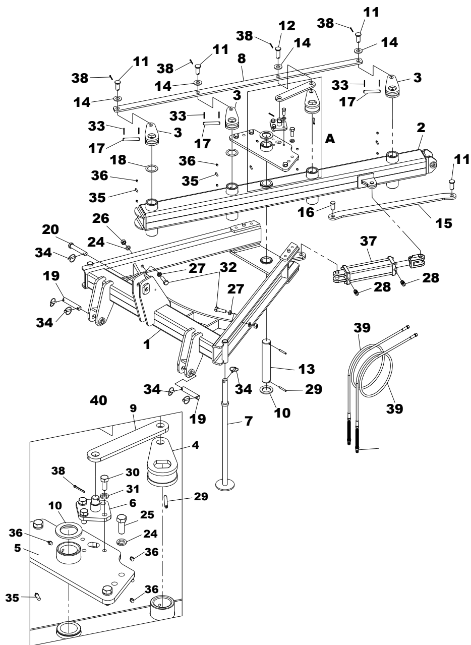
DETALLE A
